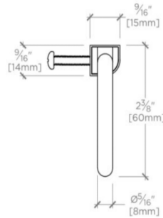
SIDE VIEW SCALE: 6"=1'-0"
